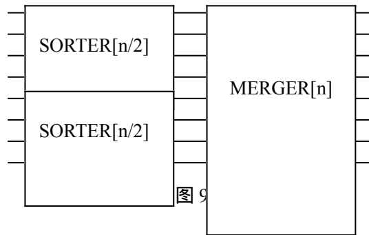
图 8 为 MERGER[n] 的一般构造方法以及 n=8 时的具体情况。 SORTER[n] 的构造方法即如图 9 所示。
