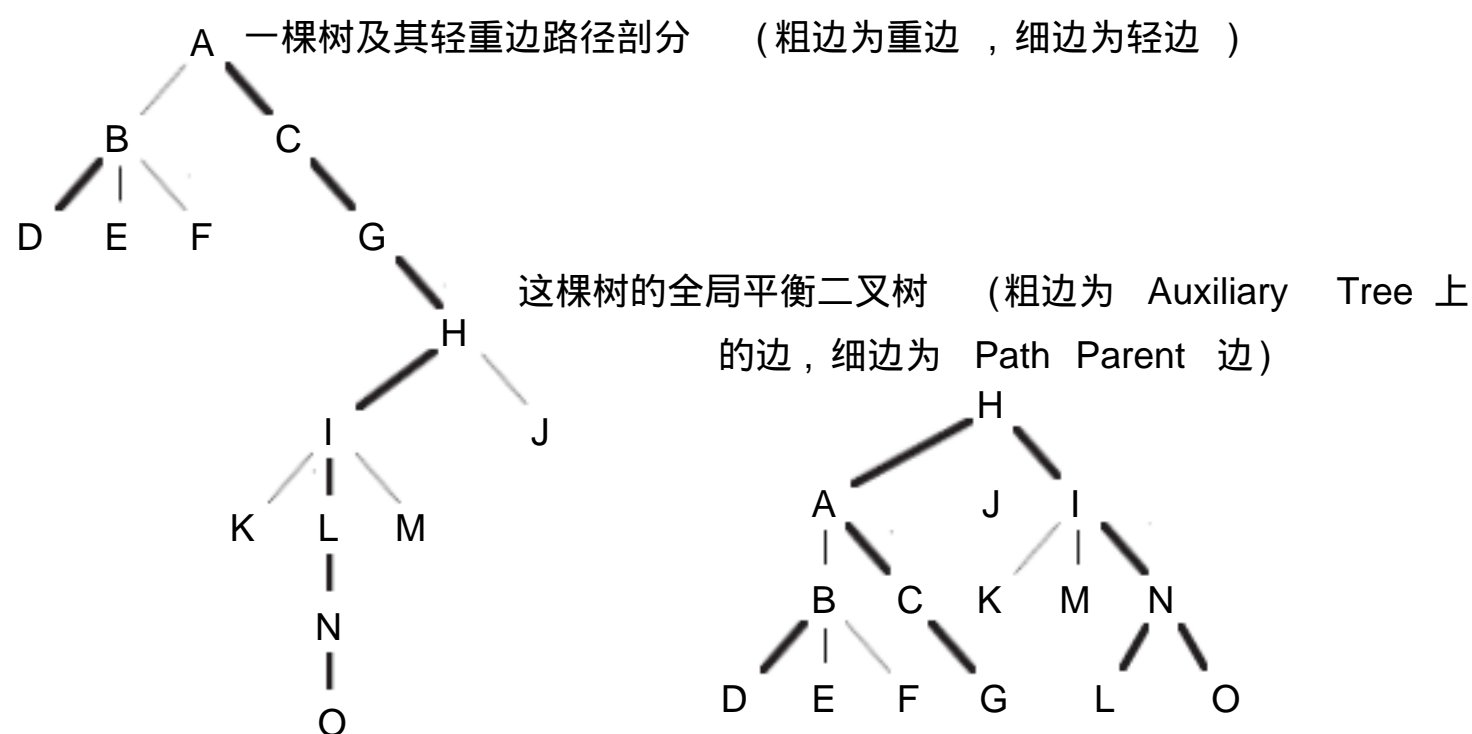
图 2: 一棵树及其全局平衡二叉树
